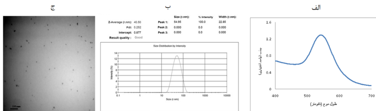
شکل ۱: طیف SPR، طیف DLS و عکس میکروسکوپ الکترونی TEM نانو ذرات کروی شکل طلا (از راست به چپ)
