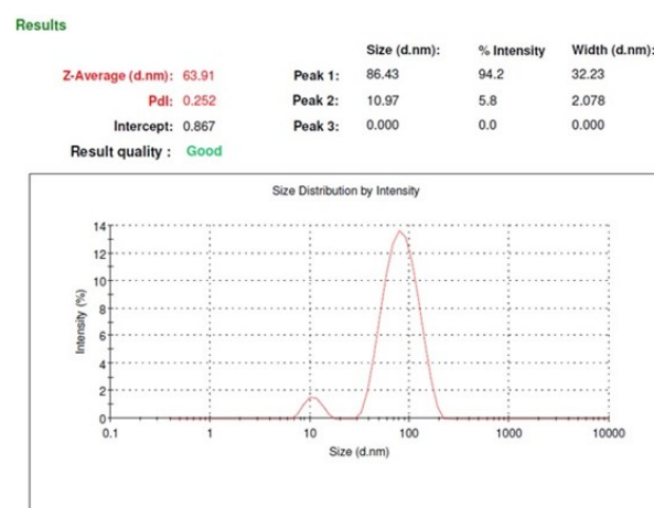
شکل ۳: طیف DLS نانو ذرات طلا در حضور آپتامر و نمک NaCl
