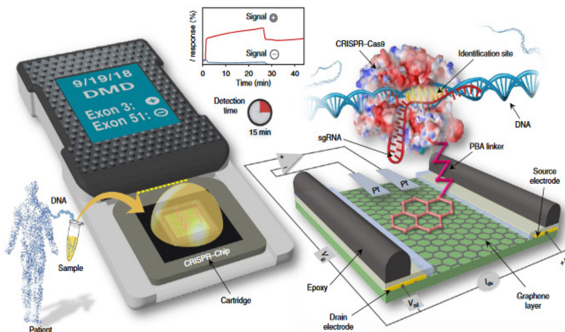
شکل ۷: کریسپر چیپ تشخیص ژن را در کمتر از ۱۵ دقیقه امکان پذیر می کند. کریسپر چیپ از توانایی هدف گیری ژن توسط Cas9-CRISPR و حساسیت gFET برای شناسایی سریع یک هدف ژنی از کل نمونه ژنومی بدون تکثیر استفاده می کند [۳۰].
