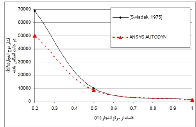
شکل ۷: مقایسه نتایج مدل رایانه‌ای (نرم‌افزار ANSYS) فشار موج انفجار نارنجک با خرجی معادل ۱۷۰ گرم TNT در حالت آزاد و انعکاس یافته با مقادیر آزمایشگاهی Swisdak [۳۱] و Petes [۳۲].
