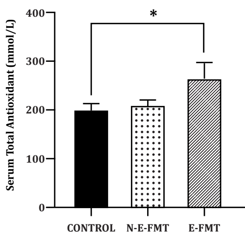
شکل ۲) ظرفیت تام آنتی‌اکسیدانی سرم موش‌های نر. در گروه دست‌نخورده، موش‌های این گروه هیچ درمانی دریافت نکردند؛ گروه کنترل، موش‌ها تحت درمان سه ماهه با CUMS قرار گرفتند؛ گروه N-E-FMT، موش‌ها در معرض CUMS قرار گرفتند و پس از تخلیه میکروبیوتای روده، دو هفته FMT دریافت کردند؛ گروه E-FMT، موش‌ها در معرض CUMS قرار گرفتند و پس از تخلیه میکروبیوتای روده، دو هفته FMT از موش‌های آموزش‌دیده ورزشی دریافت کردند. داده‌ها به صورت میانگین \pm میانگین استاندارد (SEM) ارائه شده‌اند. (*) p < 0.05 .
