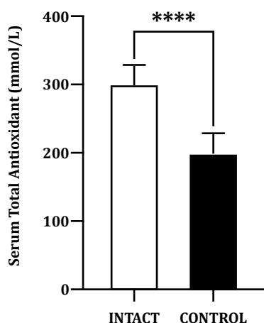
شکل ۱) ظرفیت تام آنتی‌اکسیدانی سرم موش‌های نر. موش‌های گروه کنترل هیچ درمانی دریافت نکردند. در گروه‌های دیگر، موش‌ها تحت اعمال CUMS به مدت سه ماه قرار گرفتند. داده‌ها به صورت میانگین \pm SEM ارائه شده‌اند. (****) p < 0.0001 .
