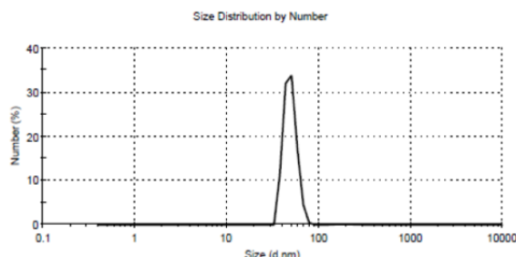
شکل ۲) اندازه‌گیری پراکنش اندازه ذرات با DLS نشان داد که پراکنش اندازه ذرات EVs جداسازی شده از خون در محدوده ۵۰ تا ۱۰۰ نانومتر است.
