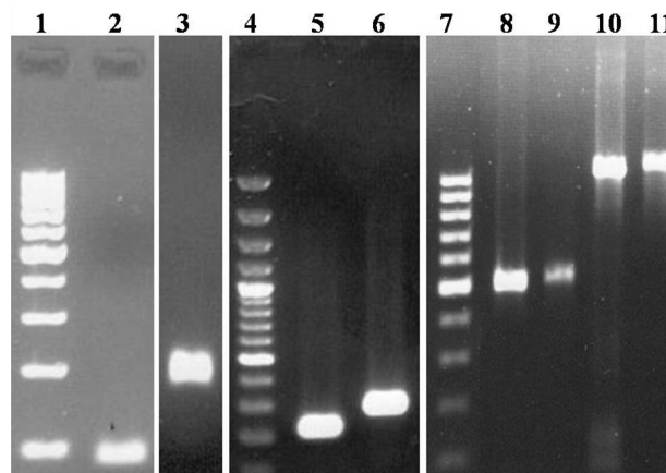
شکل ۱: آنالیز محصول PCR تکی با استفاده از الکتروفورز ژل آگارز رنگ شده با اتیدیوم بروماید. (۱ و ۴ و ۷) مارکر وزنی DNA، ۱۰۰ bp. (۲) محصول PCR تکی با پرایمرهای M3، (۳) محصول PCR تکی با پرایمرهای M4، (۵) محصول PCR تکی با پرایمرهای M1، (۶) محصول PCR تکی با پرایمرهای M2، (۸ و ۹) محصول PCR تکی با پرایمرهای M5، (۱۰ و ۱۱) محصول PCR تکی با پرایمرهای M6.
