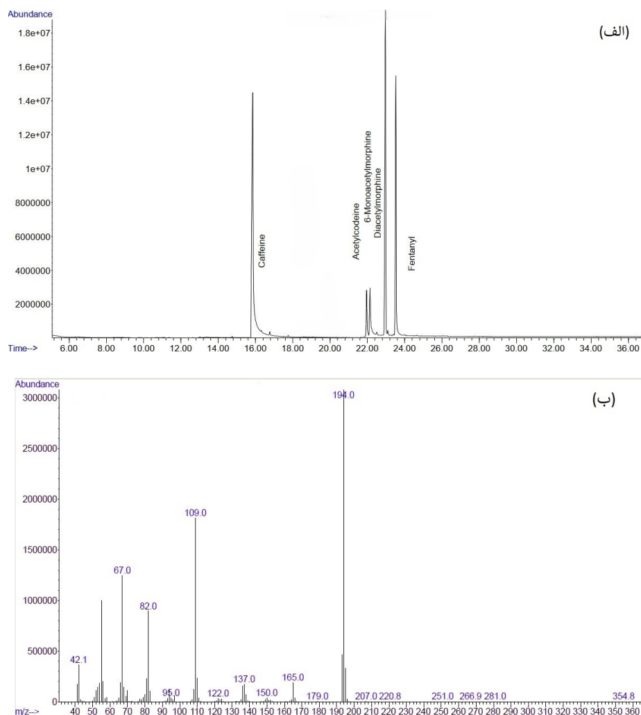
شکل ۱-الف) طیف جرمی پودر مکشوفه آنالیز شده با دستگاه کروماتوگرافی گازی-اسپکترومتری جرمی (ب) نسبت جرم به بار قطعات یونی طیف جرمی
