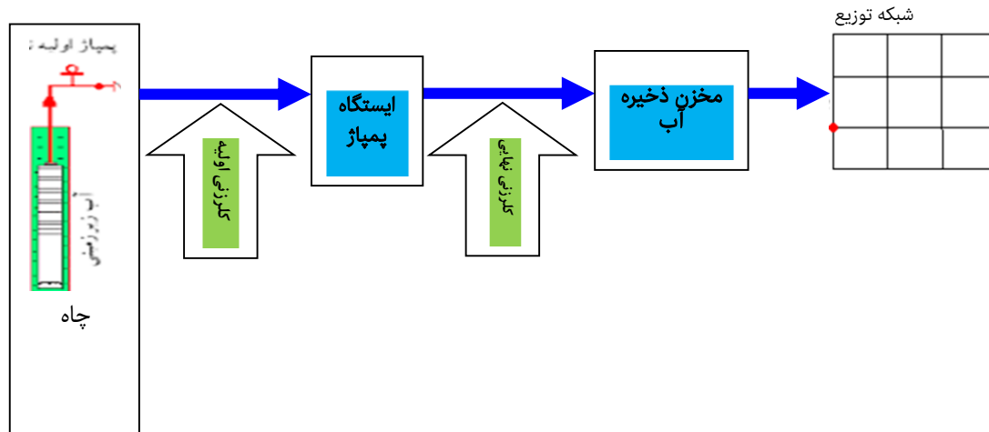
شکل ۲) فلودیگرام تأسیسات آبی شهر هشتگرد
