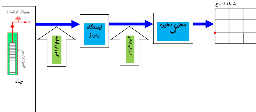
شکل ۲) فلودیاگرام تأسیسات آبی شهر هشتگرد
